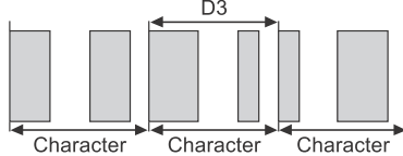
Type 3 Dimensions
